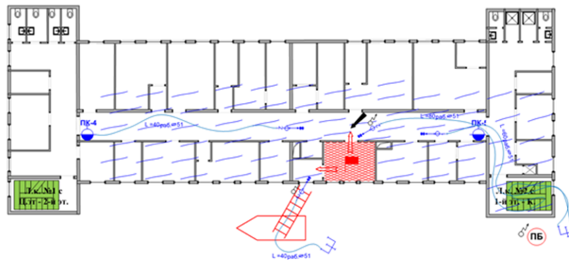
Схема подачи стволов на тушение и защиту этажей при тушении пожара на 2-ом этаже административного здания
