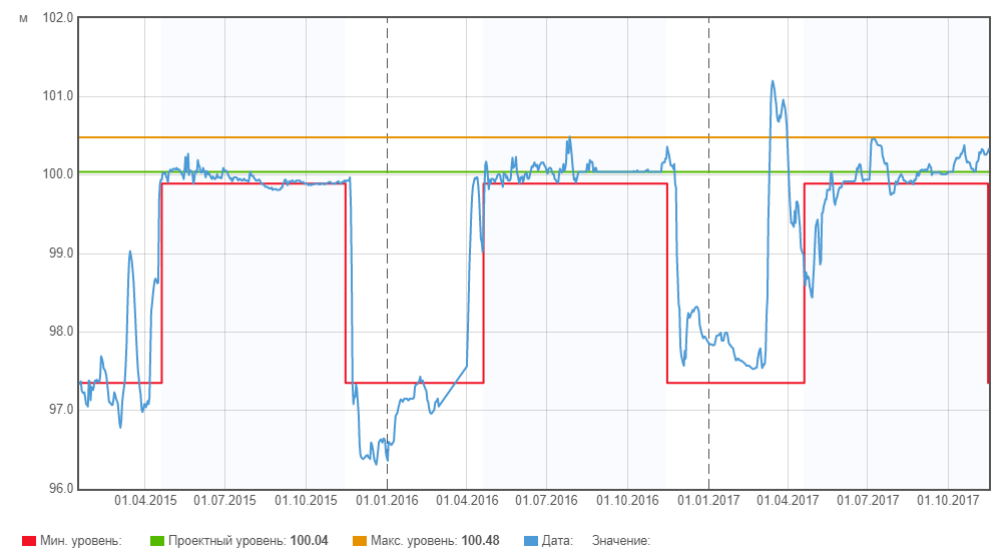
Водомерный пост
