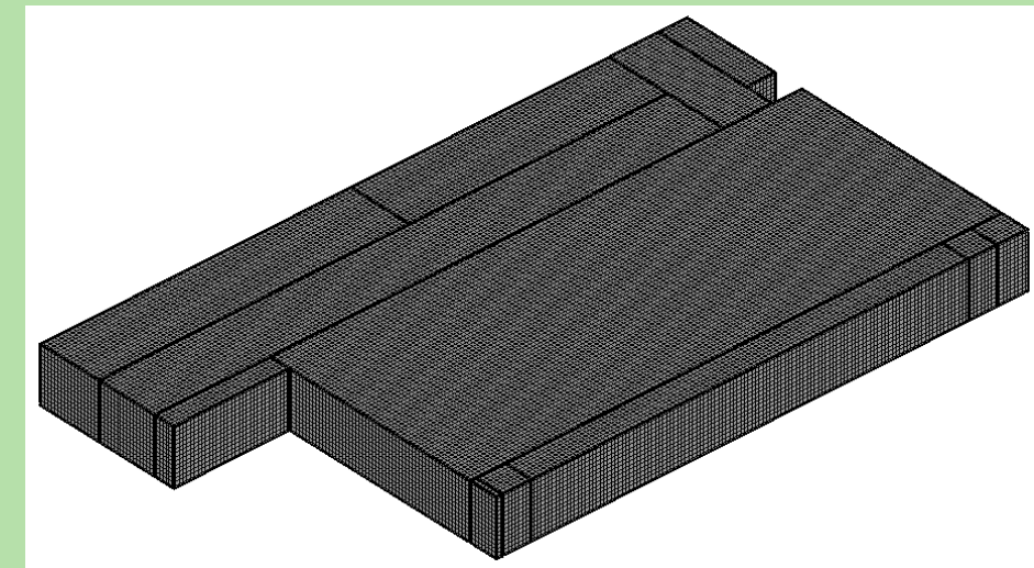
Расчетная сетка объекта
